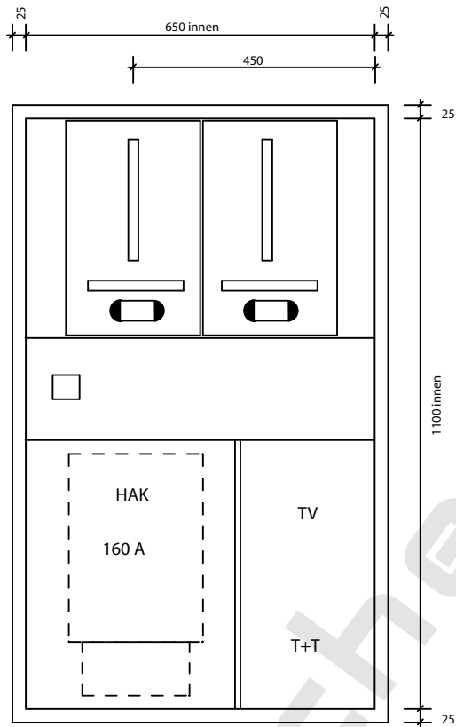
Ansicht oben SRZK 68-113 TT/TV
