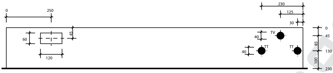
Ansicht oben SRZK 168-73 TT/TV
