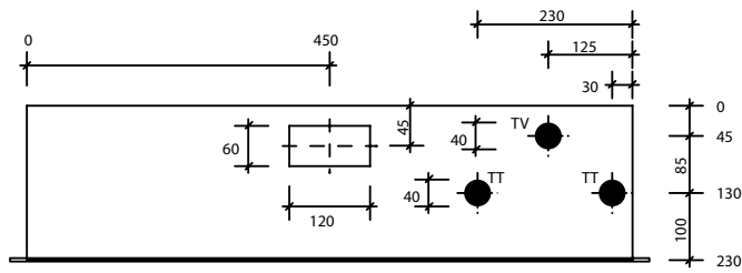
Ansicht oben SRZK 93-88 TT/TV
