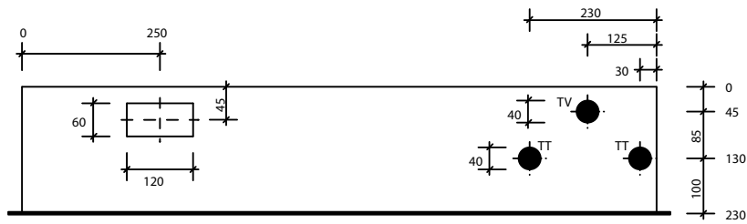
Ansicht oben SRZK 118-108 TT/TV
