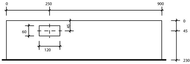
Ansicht oben SRZK 93-73
