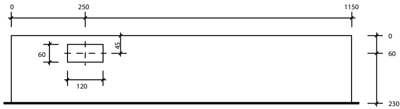
Ansicht oben SRZK 118-73
