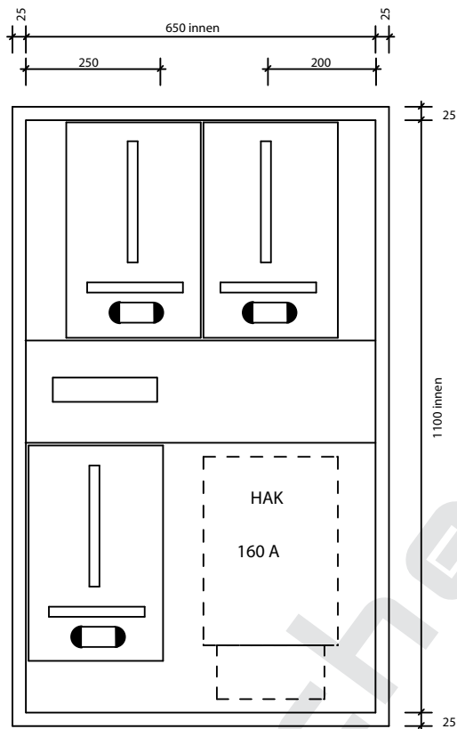
Ansicht oben SRZK 68-113
