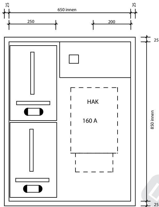
Ansicht oben SRZK 68-88
