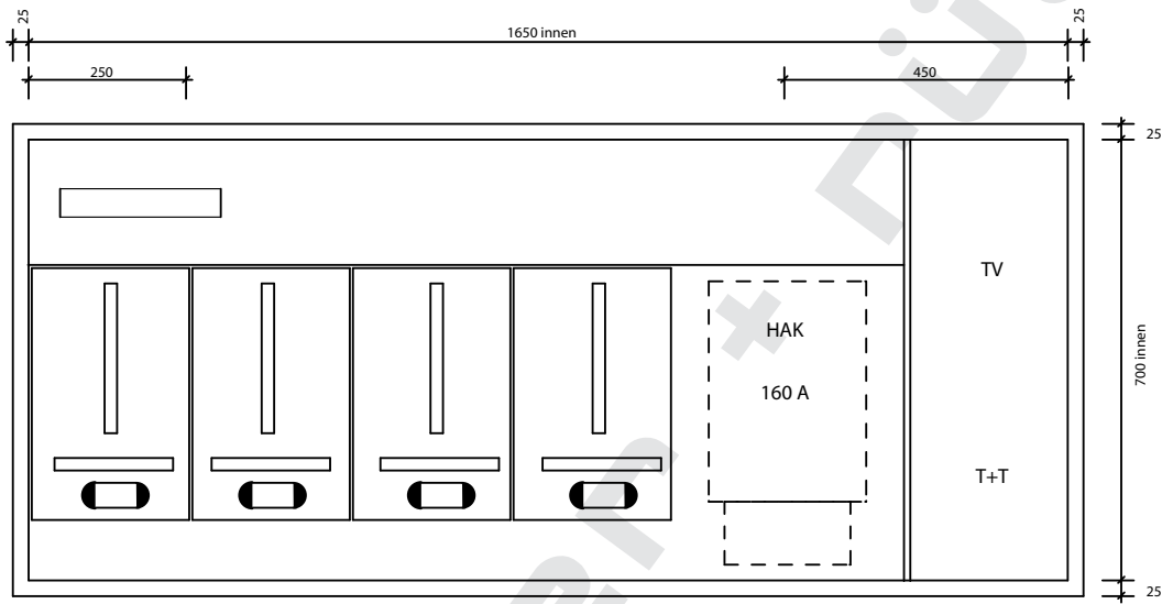
Ansicht oben SRZK 168-73 TT/TV
