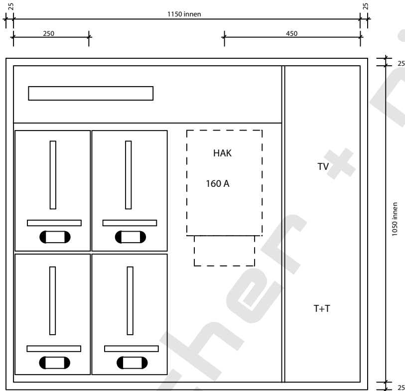
Ansicht oben SRZK 118-108 TT/TV
