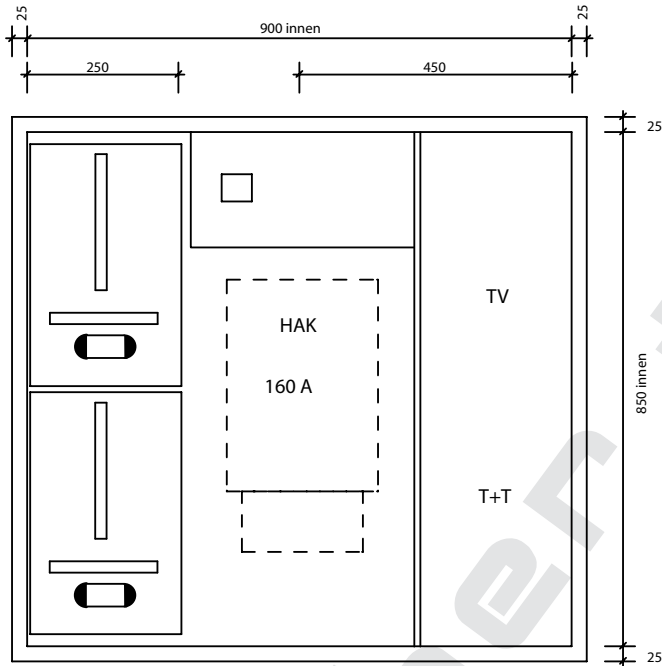
Ansicht oben SRZK 93-88 TT/TV
