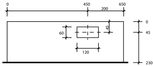
Ansicht oben SRZK 68-88
