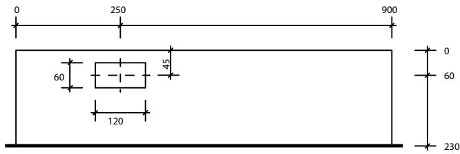
Ansicht oben SRZK 93-108
