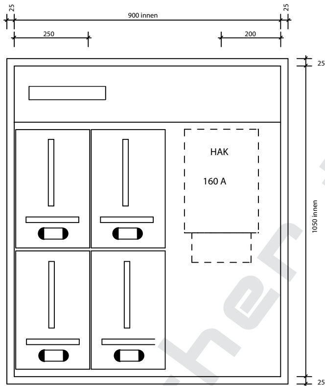
Ansicht oben SRZK 93-108
