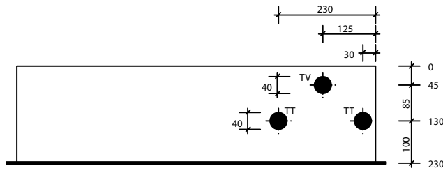
Ansicht oben SRZK 88-113 TT/TV
