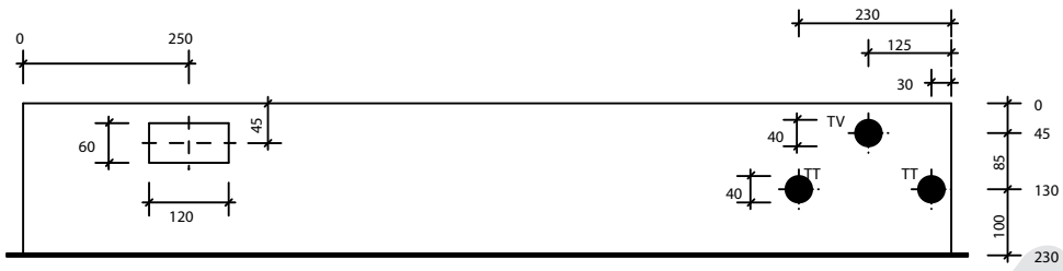
Ansicht oben SRZK 143-73 TT/TV
